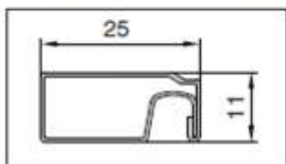
Řez profilem 25 mm
